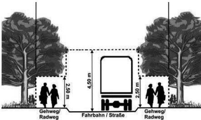
Abb.: Das Lichtraumprofil an öffentlichen Straßen und Gehwegen.
